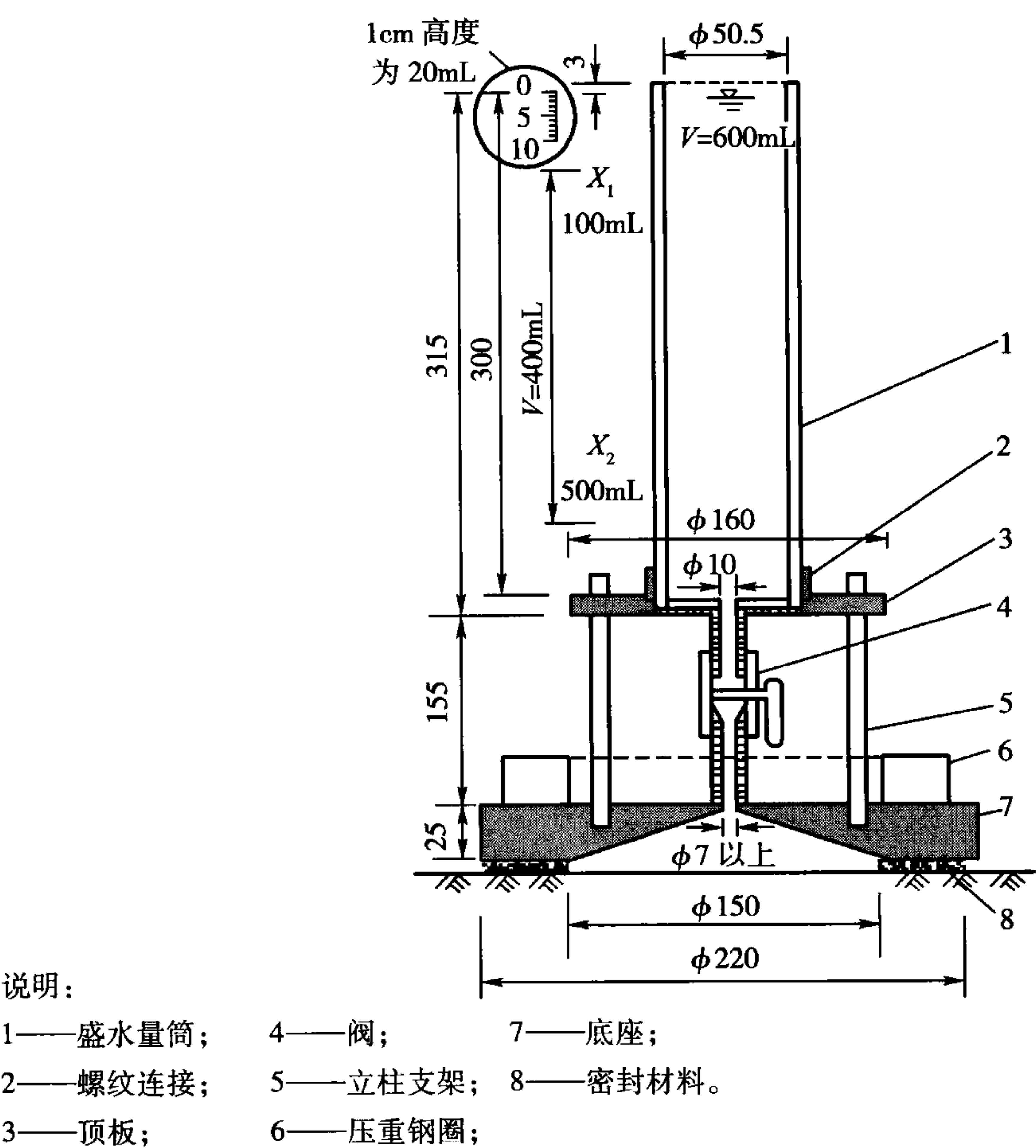
图 1 渗水仪主要结构示意图
